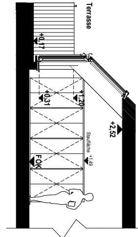
Schnitt 2
